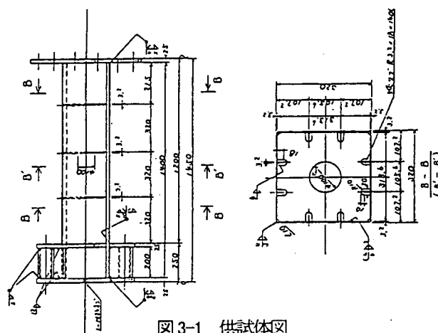
図3-1 供試体図
