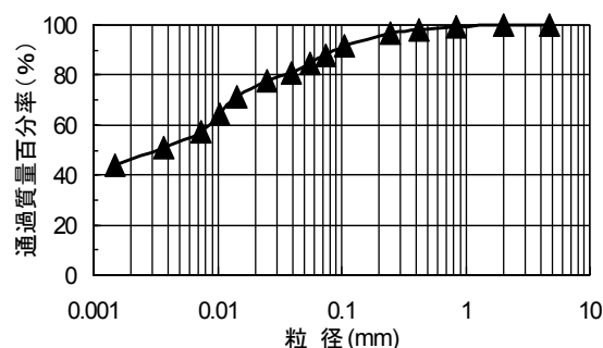
圖-1 粒徑加積曲線
