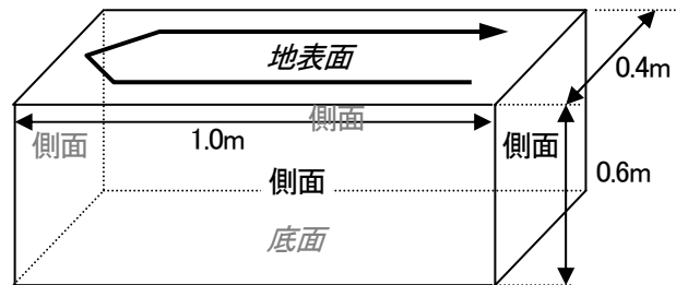
図-5 転圧回数 1 回(1 往復)
