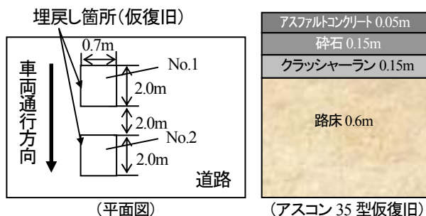
図-16 埋戻しの状況
