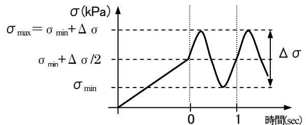
図-7 応力の載荷方法 11)
