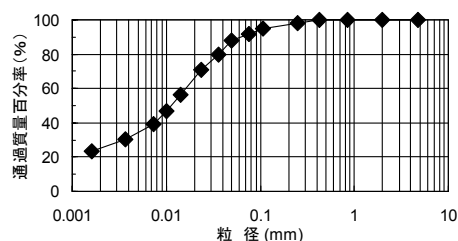
図-17 粒径加積曲線
