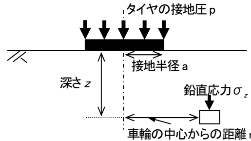
図-13 タイヤの接地圧および路床における鉛直応力
