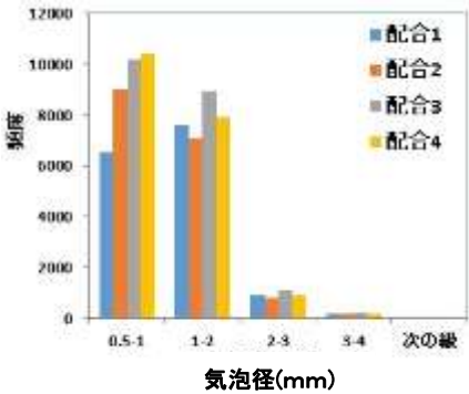
図-4 気泡ヒストグラム
