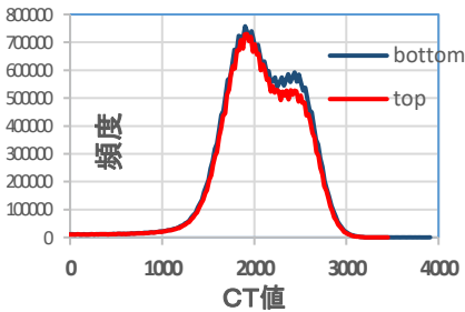
図-5 均質性ヒストグラム
