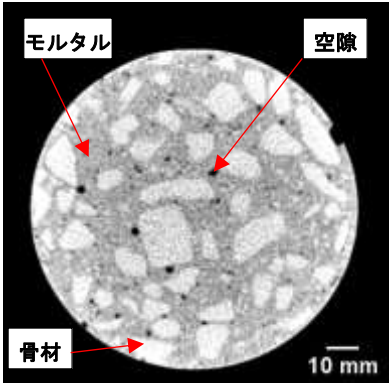
図-3 CT 断面画像
