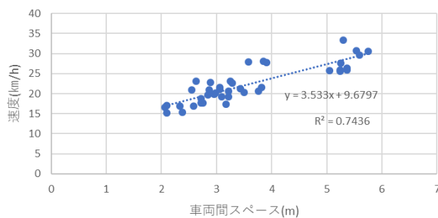
図-4 車両間スペースと速度の関係
