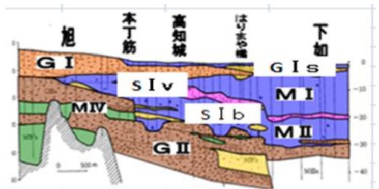
図-3 高知市周辺地盤縦断面図
