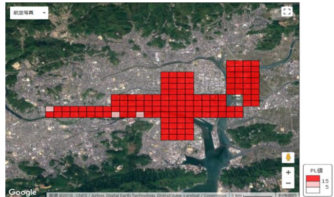
図-4 高知市地盤液状化分布図
