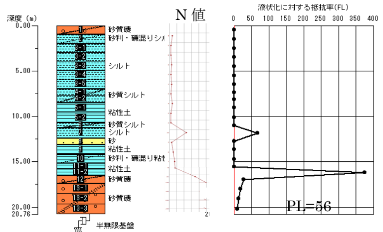
図-2 国分川流域解析例
