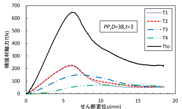
図-5 補強材軸力 T_i とせん断変位 u の関係
