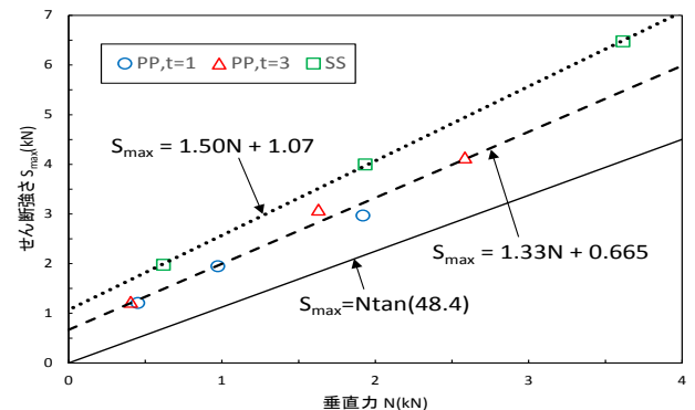
図-6 せん断力最大値 S_{\max} と垂直力 N の関係
