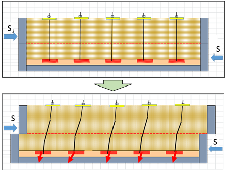
図-1 補強斜面模型実験の概念図
