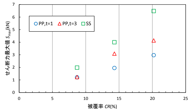
図-4 せん断力最大値 S_{\max} と被覆率 CR の関係
