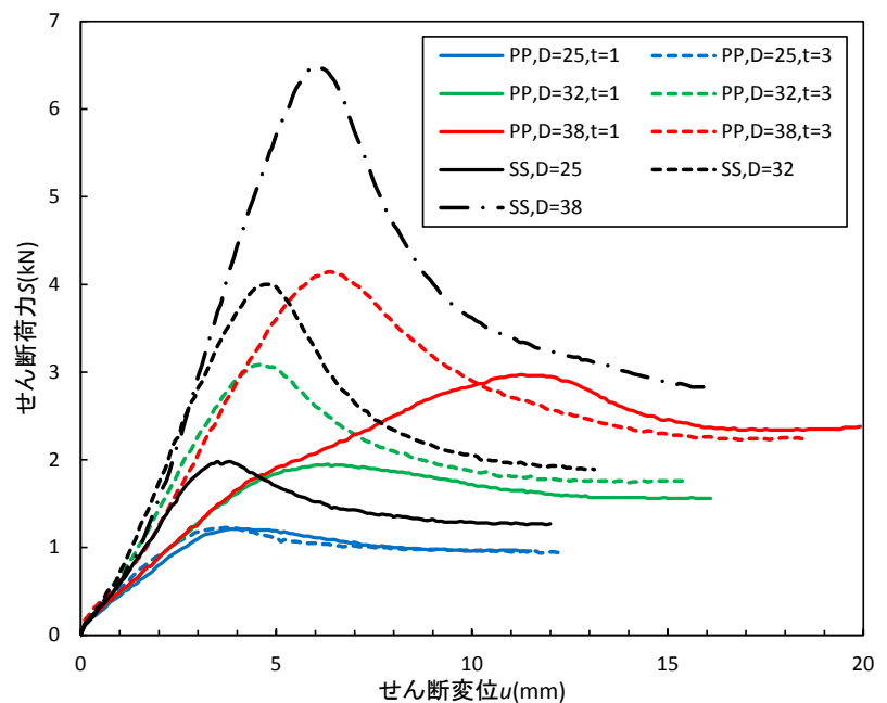
図-3 せん断力 S とせん断変位 u の関係
