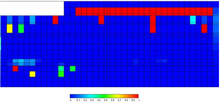
図 7 過剰間隙⽔圧比(上ノ加江地区)
