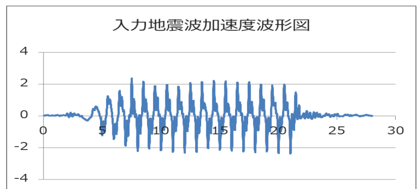
図3 入力地震波（遠心模型実験）
