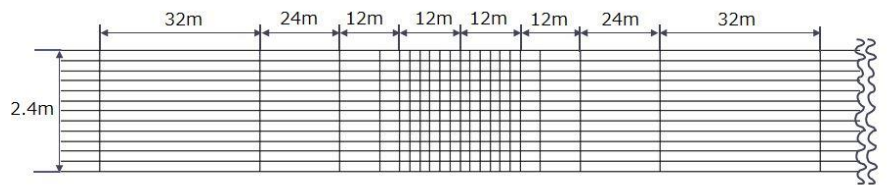
図1 動的遠心模型実験モデル
