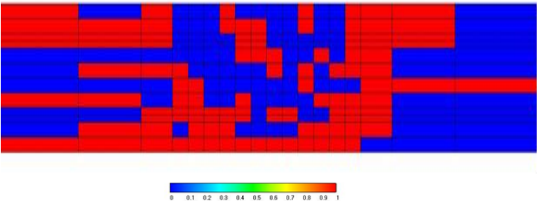
図 6 過剰間隙⽔圧比(遠心模型実験)
