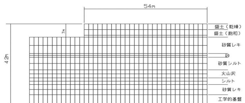
図2 上ノ加江地区の解析モデル
