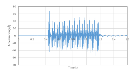
Fig.3: 改善後 (sin 波 振動数 15Hz 変位 1.0mm )
