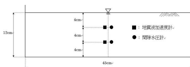
Fig.4: 実験模型
