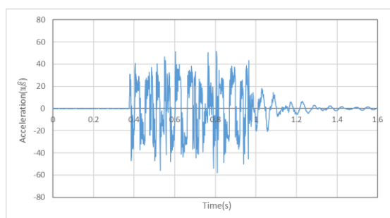
Fig.2: 改善前 (sin 波 振動数 15Hz 変位 1.0mm )
