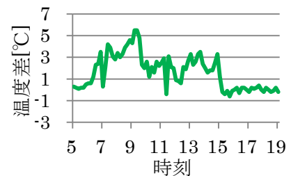
図 5. 新居浜市と K 氏宅の緑の カーテンの冷却温度の差
