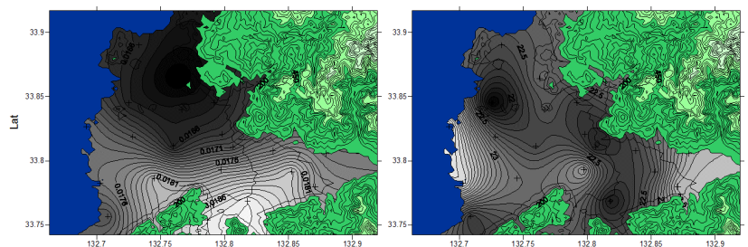
図-2 水蒸気の空間分布 (左：シミュレーション，右：現地観測)
