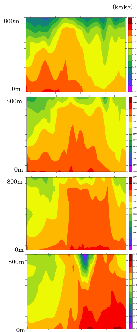
図-3 図-1AA'鉛直断面における水蒸気混合比(kg/kg)鉛直分布（上から11時, 12時, 13時, 14時）
