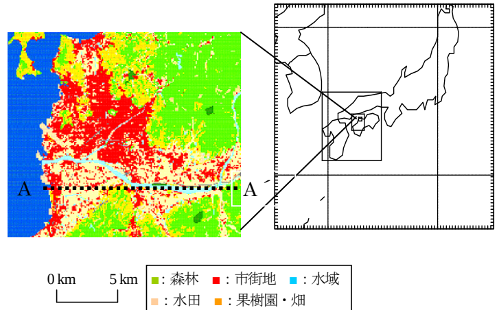
図-1 計算領域および松山平野における土地利用状況
