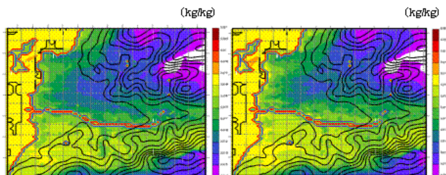
図-4 松山平野における10時の地上2mの水蒸気混合比(kg/kg)水平分布 (土地利用: 左図2006年, 右図1987年)
