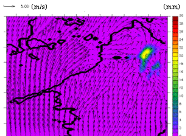
図-3 16 時における 1 時間降水量分布および地上 10m の風ベクトル
