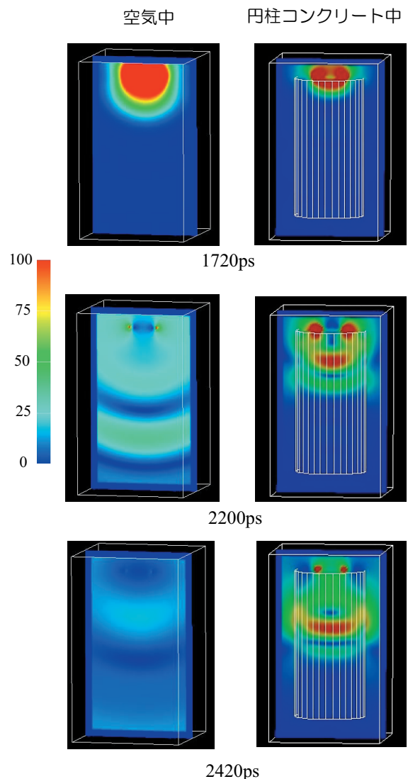
図-4 電磁波伝搬のスナップショット (左: 空気中, 右: 円柱コンクリート中の電場の絶対値)
