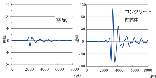
図-3 空気中と円柱コンクリート供試体中の電磁波伝搬の波形比較 [計測波形 (上) と解析波形 (下)]
