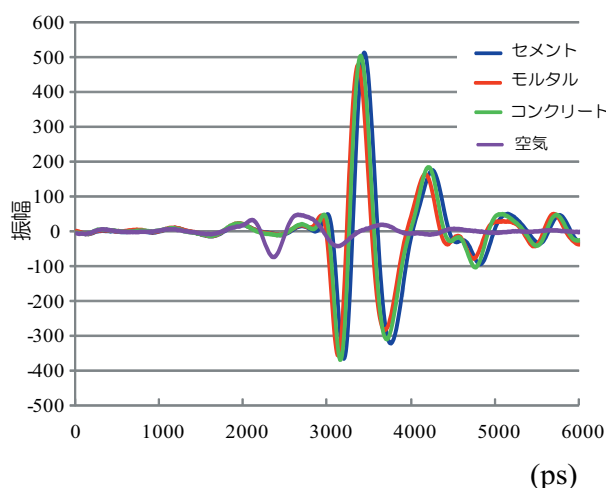
図-1 セメントペースト、モルタル、コンクリート供試体、および空气中を伝搬する電磁波の波形
