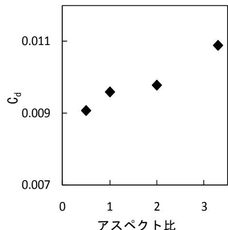
図-2 抵抗係数 C_d の比較
