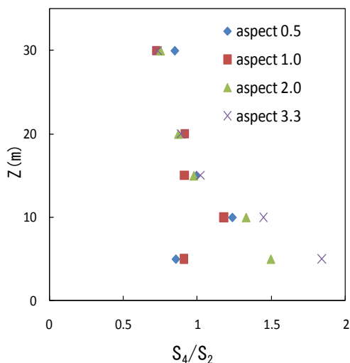
図-5 S_4/S_2 の比較
