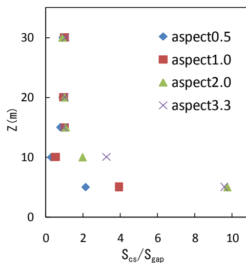
図-4 S_{cs}/S_{gap} の比較
