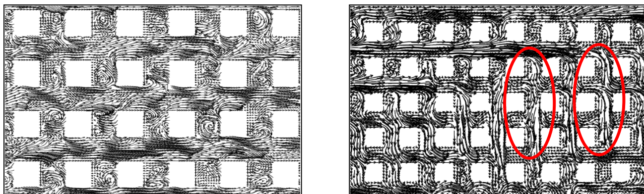
図-3 地上 1 m での瞬間風速ベクトル分布 〈(a)アスペクト比 1.0 , (b)アスペクト比 3.3 〉
