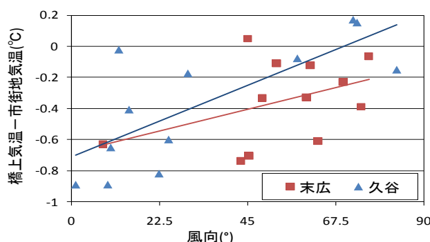
図-8 瀬切れ状態における 1 時間毎の橋上気温と風向の関係
