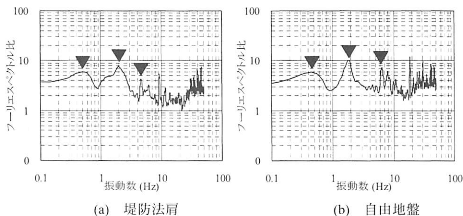
図-4 H/V フーリエスペクトル比（堤防軸直角方向）
