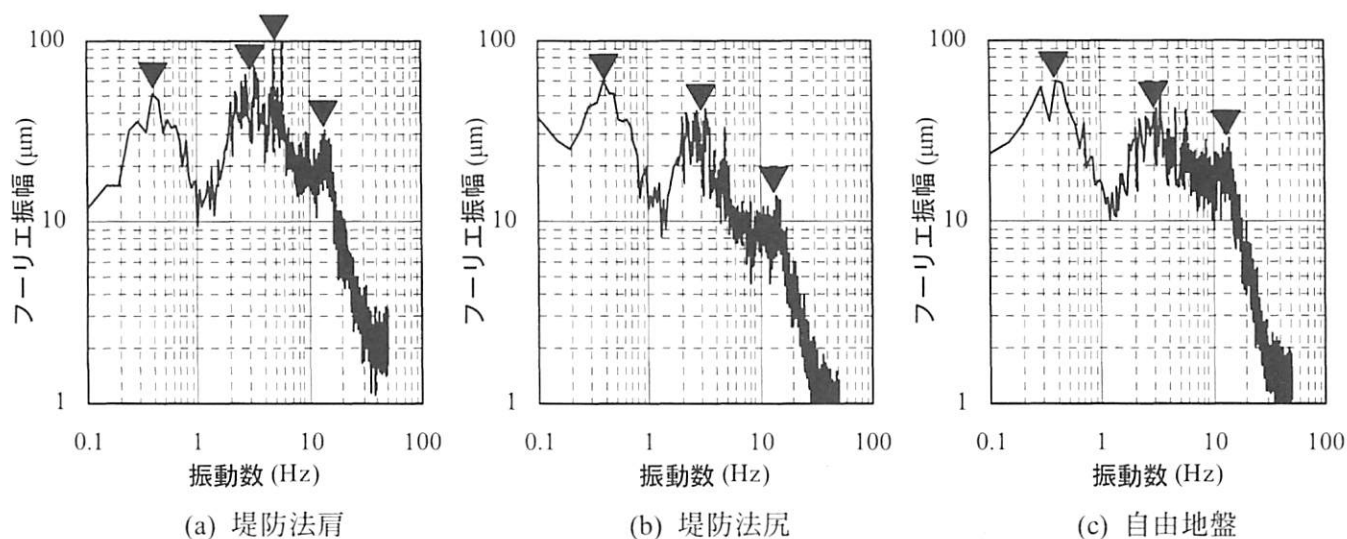
図-3 フーリエスペクトル（水平動：堤防軸直角方向）
