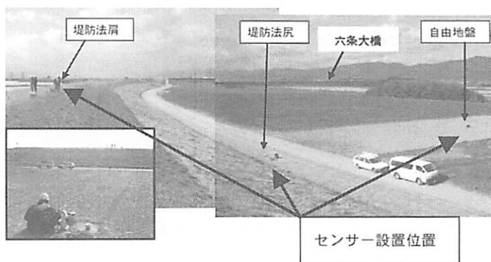
図-2 Y-5 地点における常時微動測定の様子
