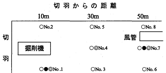
図1 粉じん測定機器配置図
