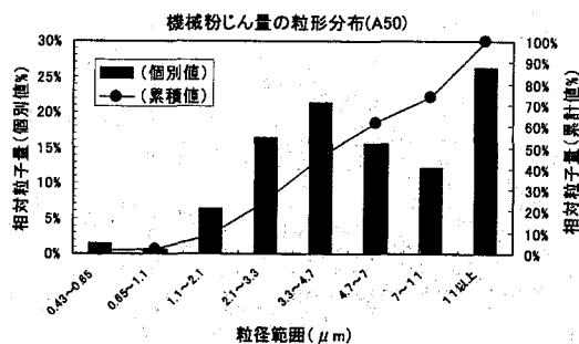
図4 コンクリート 20MPa(送風量 1,000m 3 /min, 散水無し)
