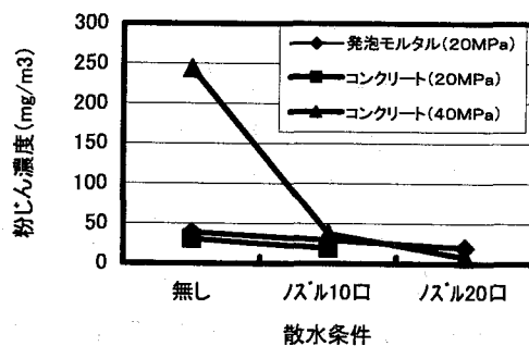
図3 散水量と粉じん濃度の関係(50m地点)
