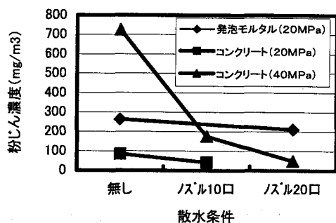
図2 散水量と粉じん濃度の関係(10m地点)
