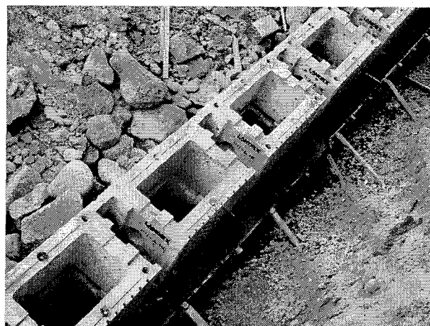
写真-3 コンクリート打設状況
