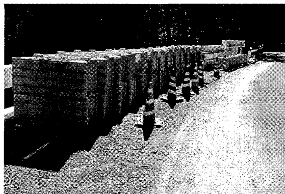
写真-2 自立型省スペース構造
