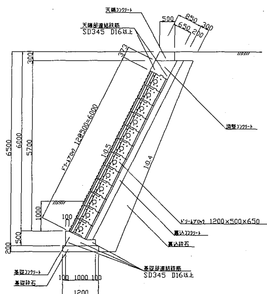
图-1 標準断面图
