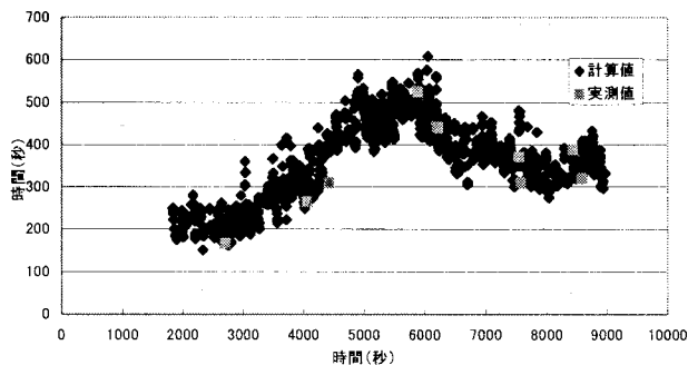
図－4 西行き旅行時間も演算値と実測値の関係
