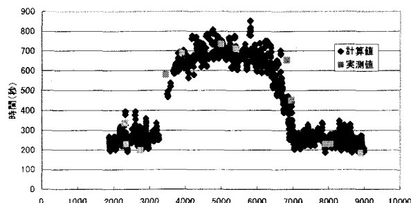
図－3 東行き旅行時間も演算値と実測値の関係
