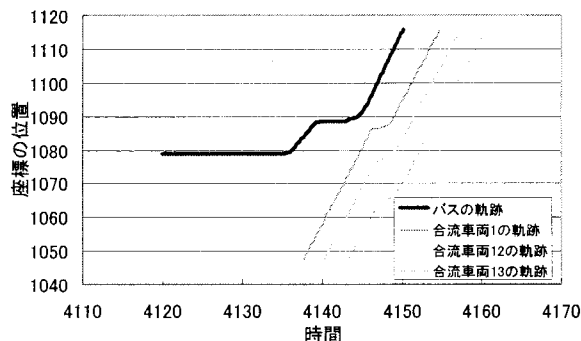
図－7 電停共有化後の車両の軌跡
