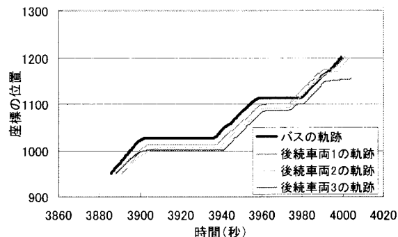
図－6 現状における車両の軌跡
