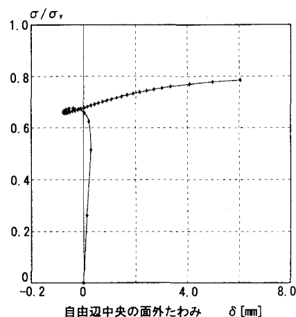
図-4 荷重-面外たわみ関係 (A1)
