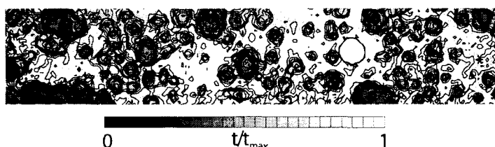
図-1 板厚等高線図(A1)
