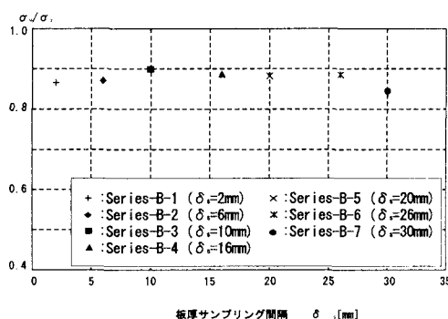
図-7 \sigma_u/\sigma_y - \delta_s 関係 (B2)
