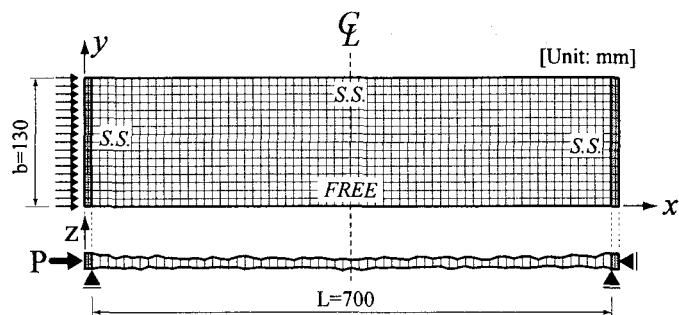
図-3 解析モデル
