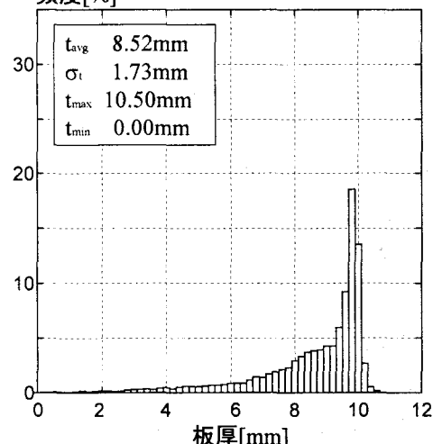
図-2 板厚ヒストグラム(A1)
