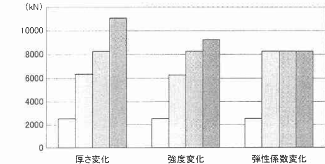
図-3 せん断耐力
