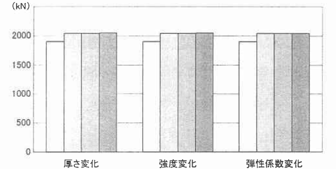
図-1 終局水平耐力
