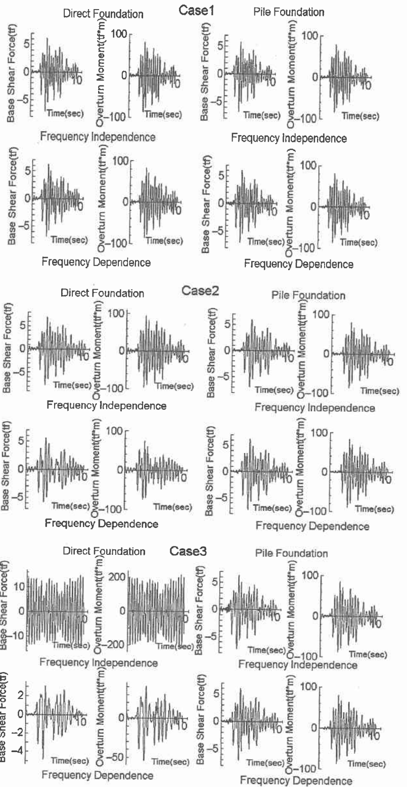
図 4 せん断力と転倒モーメントの時刻歴波形
