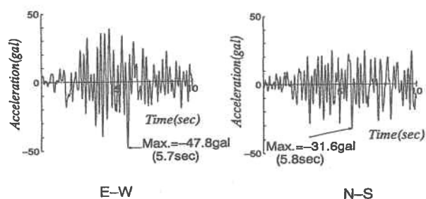
図3 基盤の地震波形
