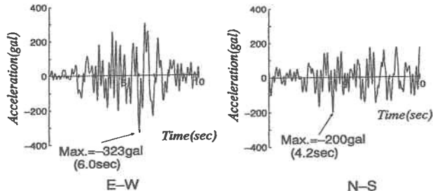
図4 地表面の波形（基盤の波形を4.2倍して入力）
