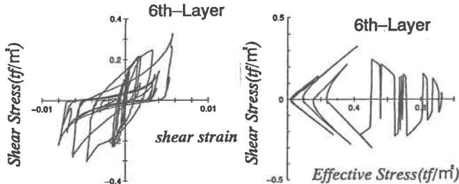
(b) 復元力特性
