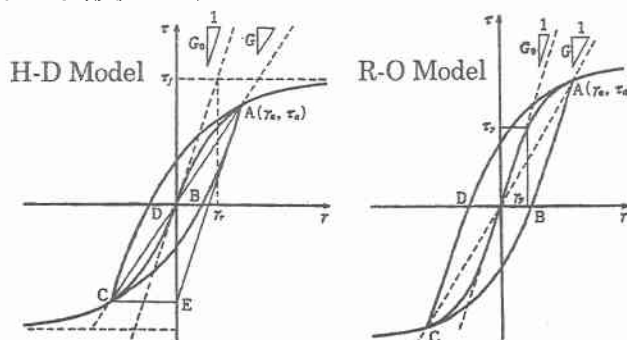
図-1 せん断応力とせん断ひずみの復元力特性曲線
