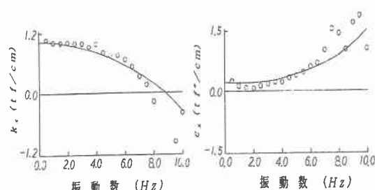
図-1.1 複素剛性の概念
