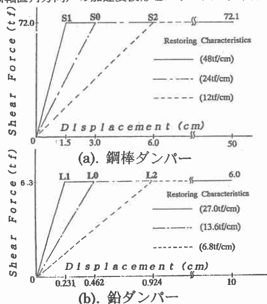
図4. (a)・(b) ダンパーの復元力特性
