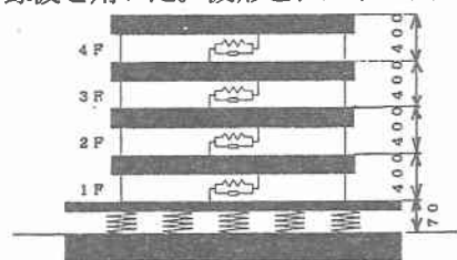
図1. 免震構造物
