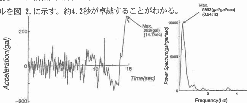
図2. 東神戸大橋（橋軸直角方向）の加速度波形とパワースペクトル
