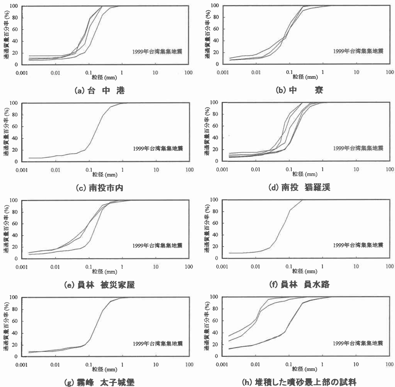
図-2 採取地点別の噴砂の粒径加積曲線
