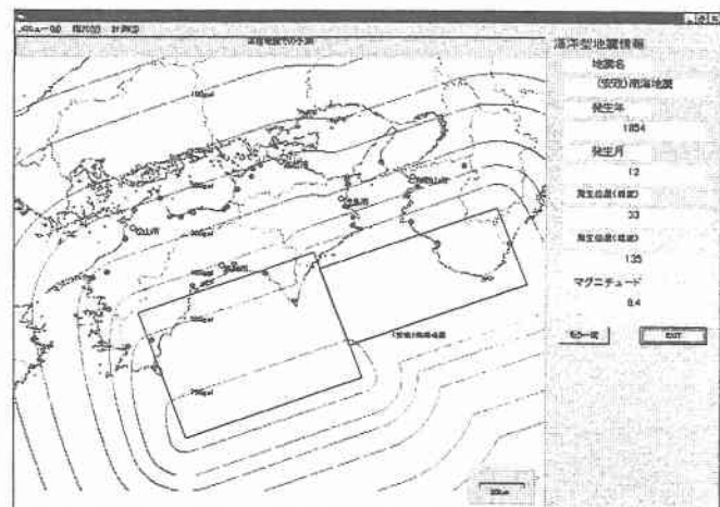
図6 最大加速度分布図(Ⅲ種地盤)
