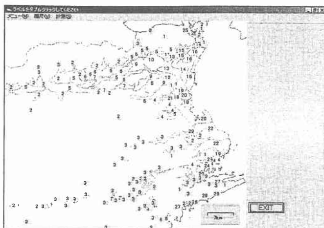
図4 地盤区分域の検索例
