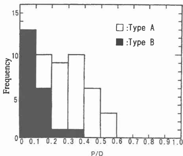
図-4 破壊タイプ別の杭頭貫入量比の頻度分布
