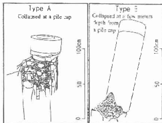
図-1 2種の典型的な杭頭破壊形態
