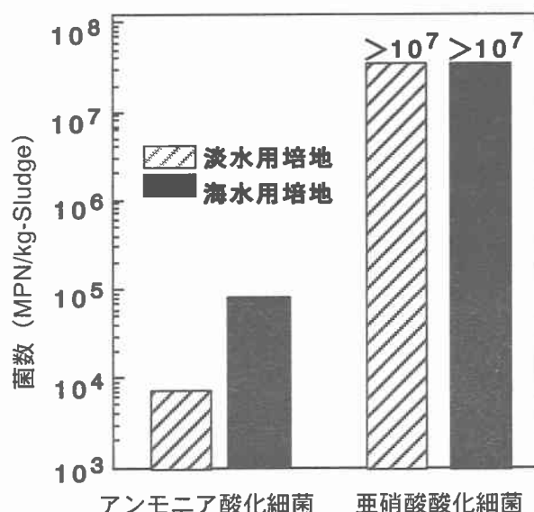
図2 海水性・淡水性培地における硝化細菌の菌数計数結果（黒瀬川感潮部底質）
