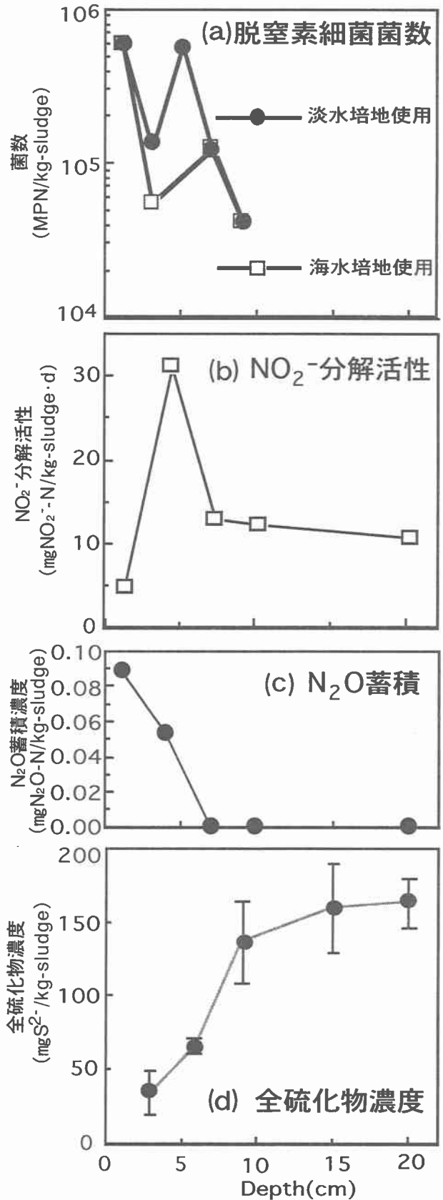
図4 窒素・硫黄化合物の深さ方向プロファイル (a) 脱窒素細菌菌数 (b) 底質の亜硝酸塩分解活性 (c) 亜酸化窒素の蓄積 ((b)図のバイアル実験終了時における) (d) 全硫化物濃度 (溶解性+固形性)
