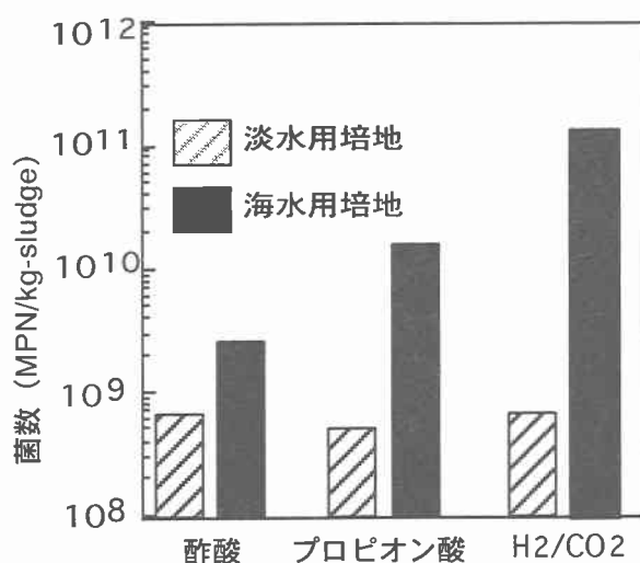
図3 海水性・淡水性培地における硫酸塩還元細菌の菌数計数結果（黒瀬川感潮部底質）
