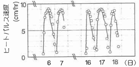
図-4 ヒートパルス速度の再現結果（8月） （—：推定値，○：実測値）
