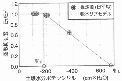
図-5 蒸散抑制度と土壌水分ポテンシャルの関係
