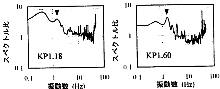
図-3 H/V スペクトル比
