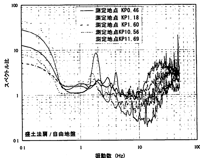
図-7 5 地点の盛土法肩/自由地盤の水平動スペクトル比
