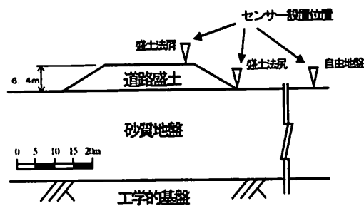
図-2 KP1.60 のセンサー設置状況
