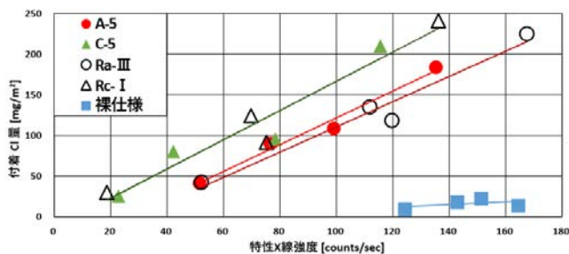
図 2 特性 X 線強度とガーゼの拭き取り法による付着 Cl 量の関係。
