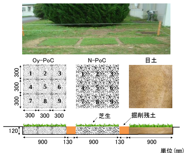
図1 実地植栽試験概略図
