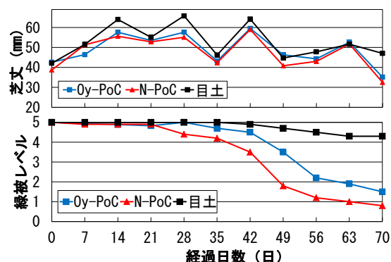
図 3 芝丈および緑被レベルの経時変化
