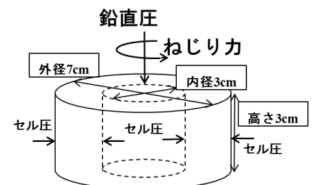
図-2 供試体に作用する力
