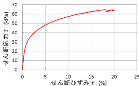
図-5 応力—ひずみ関係
