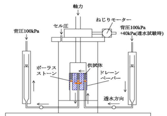
図-1 中空ねじり試験機概要
