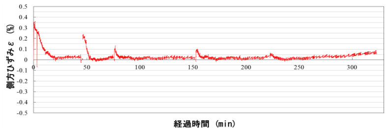
図-3 側方ひずみの経時変化
