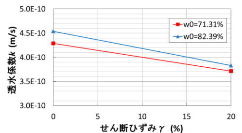
図-6 透水係数—せん断ひずみ関係
