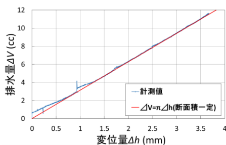
図-4 排水量—変位量関係
