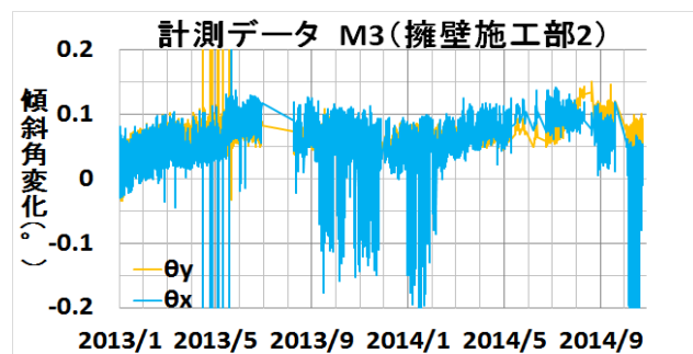
図 2 計測データ
