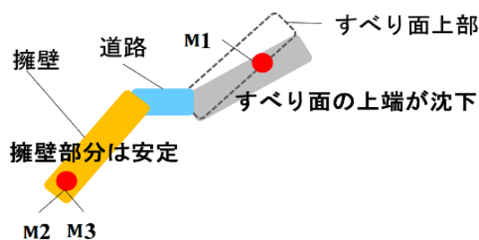
図 5 地盤の挙動
