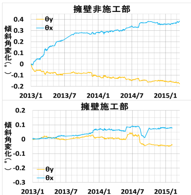
図 4 較正結果
