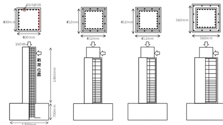
図-1 実験供試体
