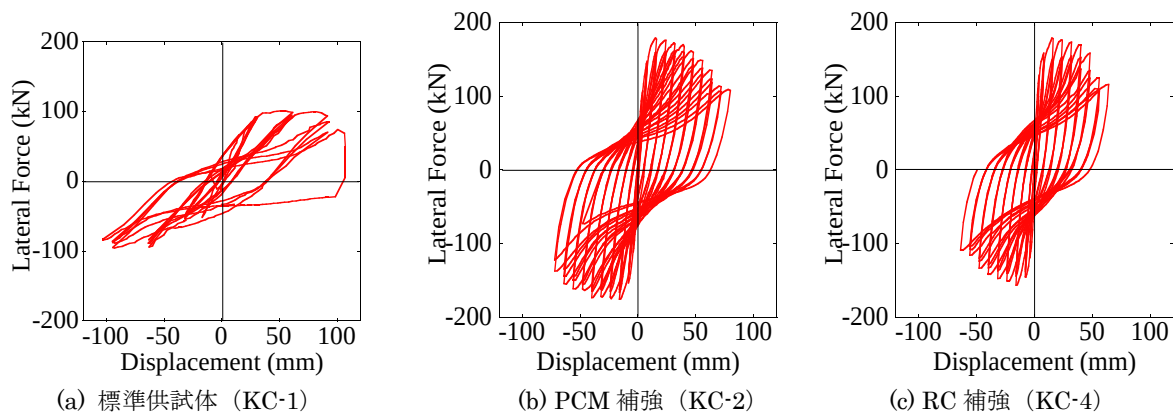
図-2 各供試体の水平力～水平変位の履歴
