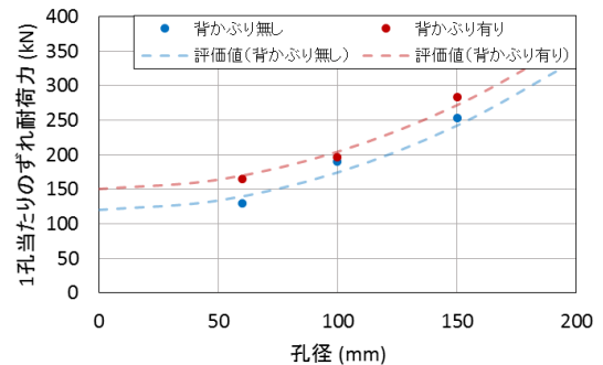
Fig.3.1 ずれ耐力力ー孔径関係
