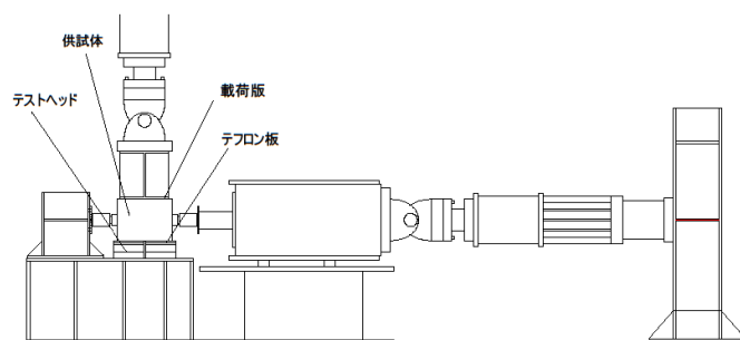
Fig. 2.2 実験装置概要
