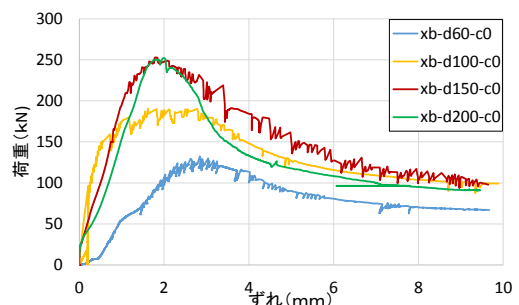
Fig.3.2 鉛直荷重ーずれ関係
