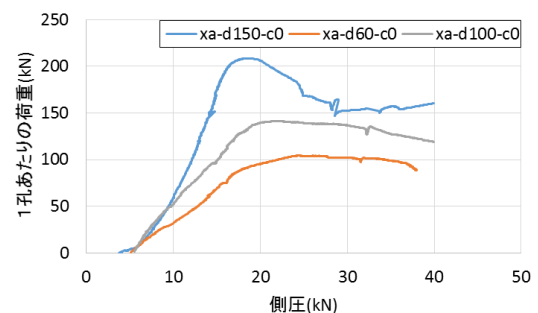
Fig.3.3 水平変位制御における鉛直荷重ー側圧関係
