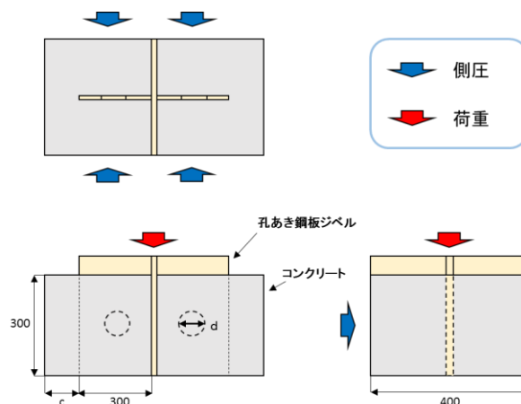
Fig. 2.1 供試体概要
