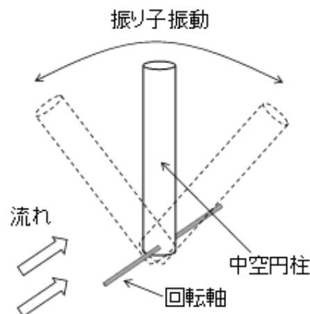
Fig. 1 Hydro-VENUS の仕組み
