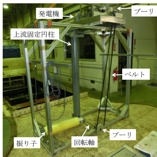
Fig. 2 Hydro-VENUS の実験装置
