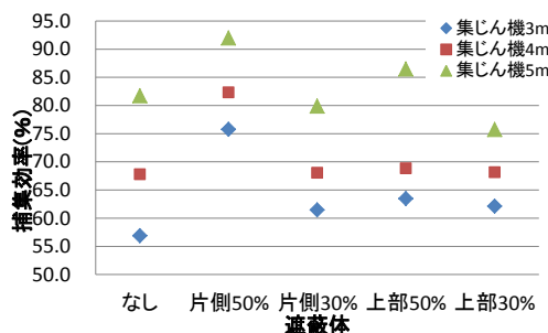
(b) 遮蔽体の面積・形状
