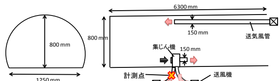
図-2 トンネル模型断面図
