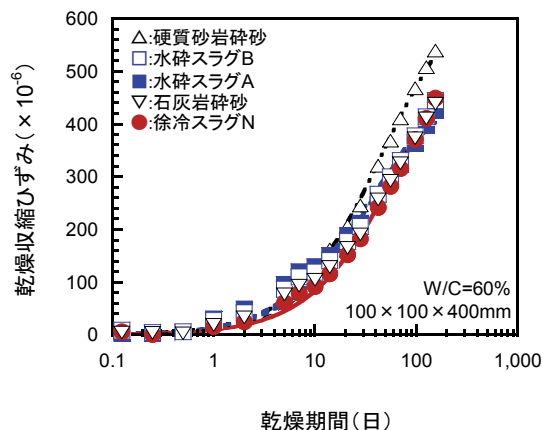
図6 乾燥収縮ひずみの測定結果(W/C:60%の場合)
