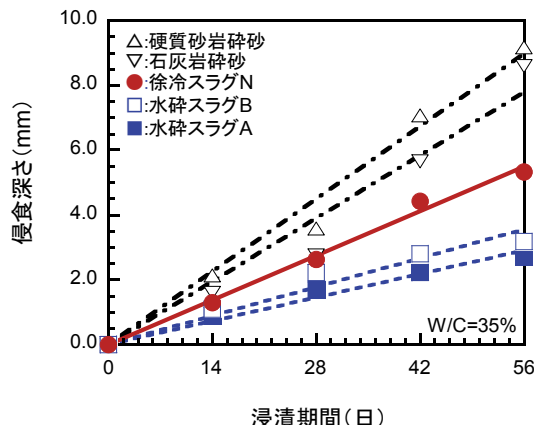
図4 耐硫酸浸漬試験の結果
