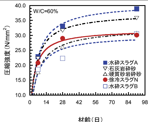
図2 圧縮強度試験の結果(W/C:60%の場合)
