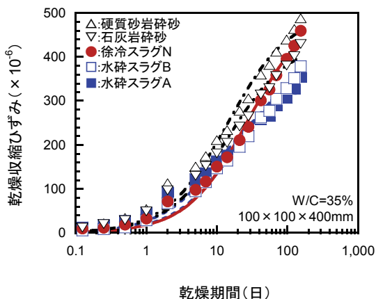
図5 乾燥収縮ひずみの測定結果(W/C:35%の場合)
