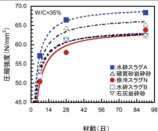
図1 圧縮強度試験の結果(W/C:35%の場合)
