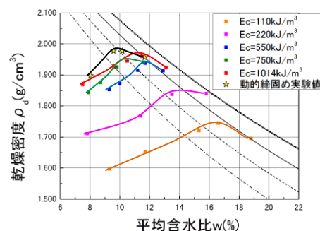
図-4 締固め曲線
