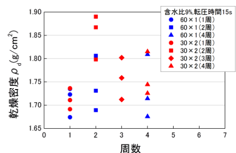
図-3 層数・転圧周数の検討
