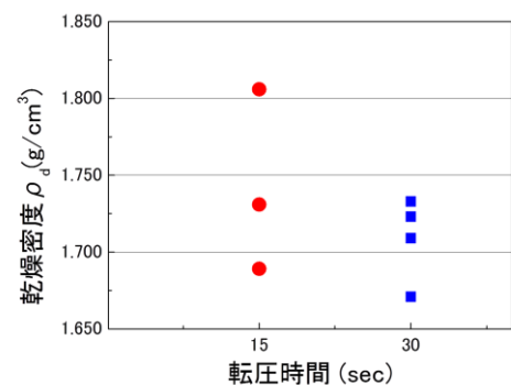
図-2 転圧時間の検討
