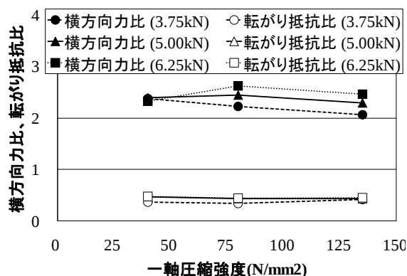
図-5 一軸圧縮強度と横方向力比、転がり抵抗比の関係
