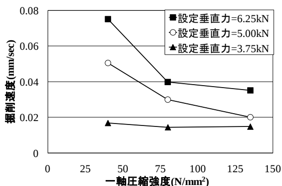
図-6 一軸圧縮強度と掘削速度の関係
