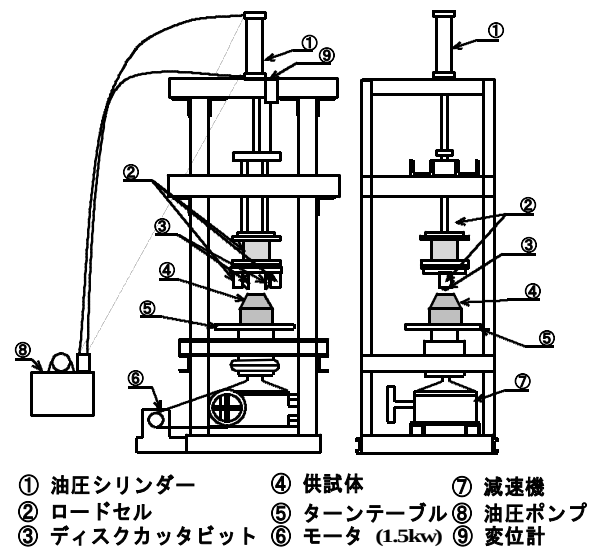
図-2 実験装置の概略図
