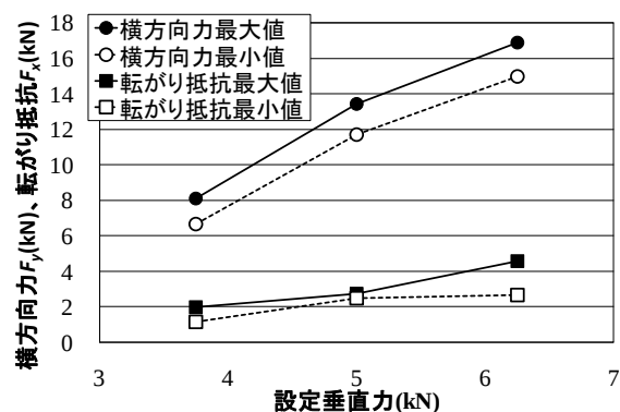
図-4 設定垂直力と各作用力最大値の関係
