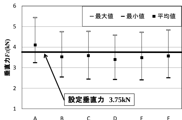
図-3 設定垂直力 3.75kN における実際の垂直力 F_z
