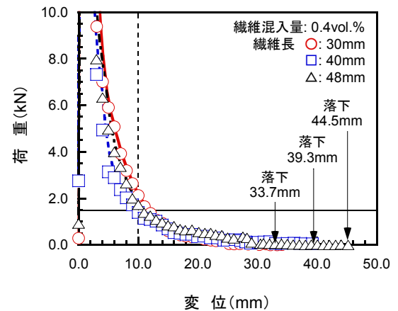
図2 繊維の長さがはく落防止効果に及ぼす影響
