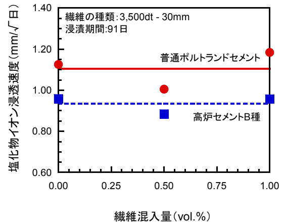
図4 繊維の混入量が塩化物イオン浸透速度に及ぼす影響
