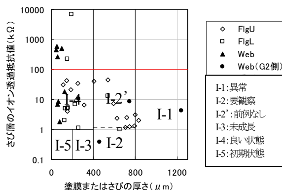
図 3 RST 法による耐候性鋼上に生成した錆の分類
