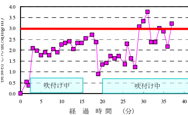
図 8 粉じん濃度 (N)
