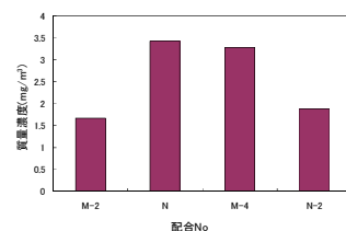
図 9 ローボリュームサンプラーを用いた各種粉じん濃度
