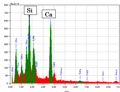
図 4 スペクトル分析
