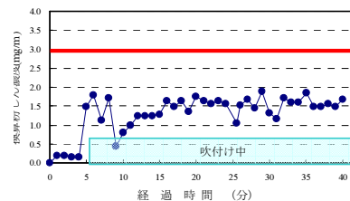
図 5 粉じん濃度 (M-2)
