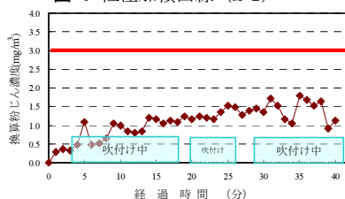
図 7 粉じん濃度 (N-2)
