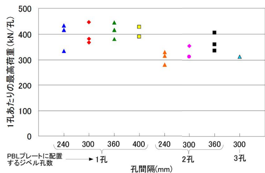
Fig.2 1孔あたりの最高荷重
