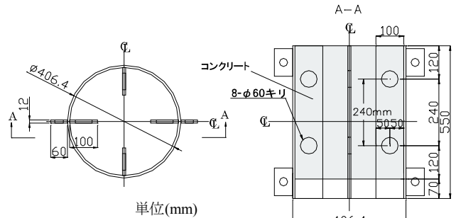
Fig.1 供試体形状例(孔間隔 240mm)
