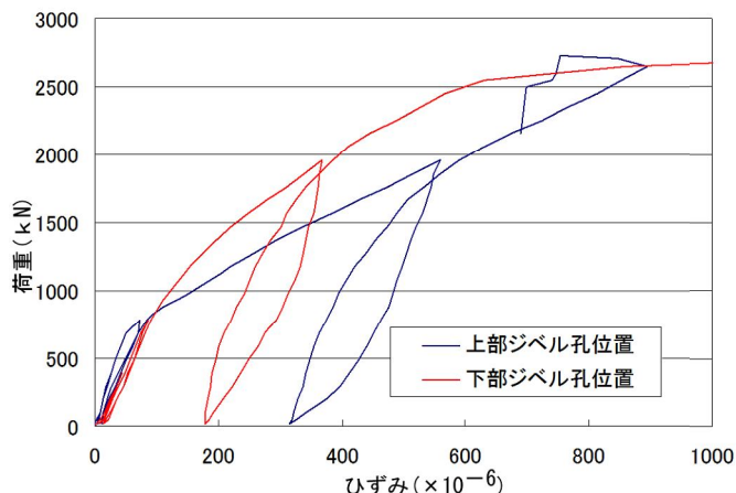
Fig.4 荷重一周方向ひずみ曲線(孔間隔 300mm)
