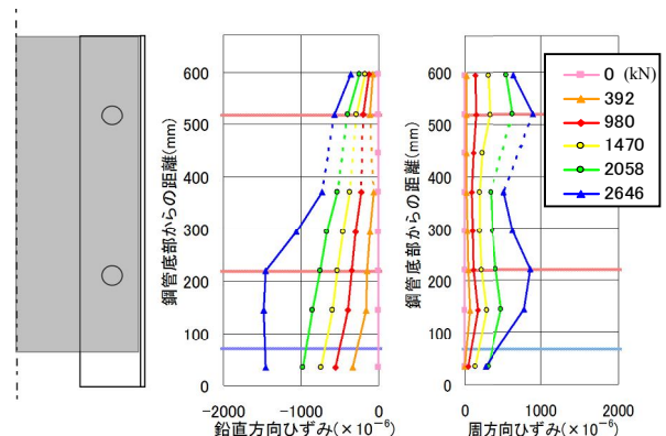
Fig.3 鋼管の軸方向でのひずみ分布(孔間隔 300mm)
