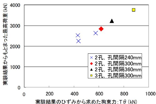
Fig.5 鋼管による拘束力と最高荷重の関係
