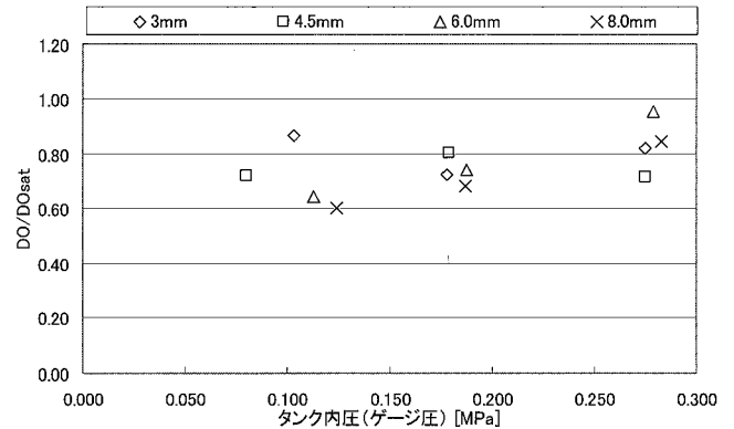
図-7 溶解率とタンク内圧の関係
