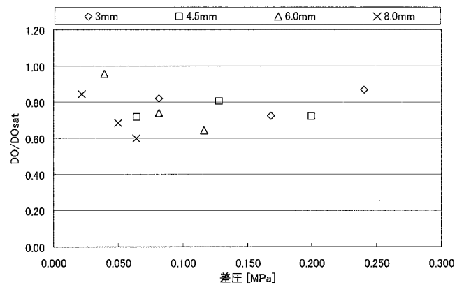
図-8 溶解率と噴射水の速度水頭の関係
