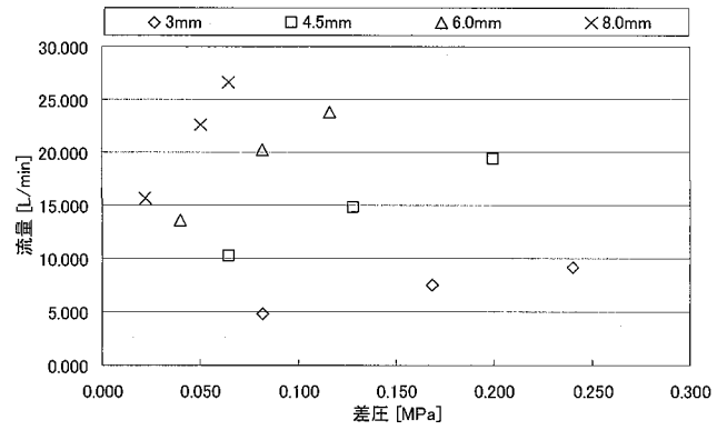
図-5 流量と差圧の関係
