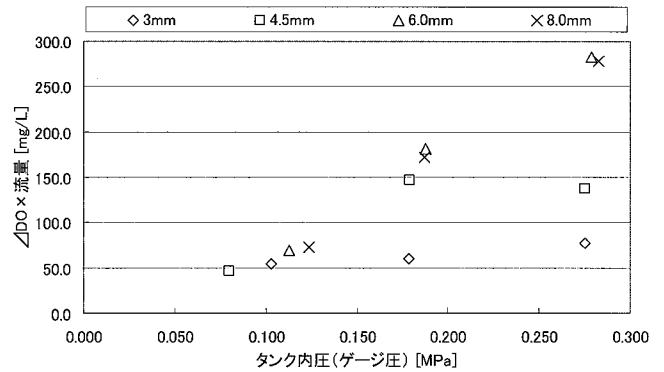
図-6 溶解能力とタンク内圧の関係
