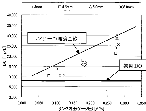
図-4 DO、ΔDO とタンク内圧の関係
