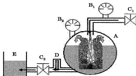
A: 耐圧タンク B1: 噴射圧 B2: タンク内圧 C1, C2: バルブ D: DO計 E: 処理水収容器
