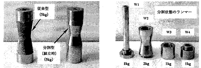
写真-1 重量可変重錘の外観
