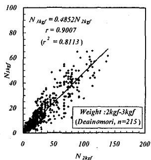
(c) N_{2kgf} と N_{3kgf} との関係
