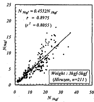
(a) N_{3kgf} と N_{5kgf} との関係
