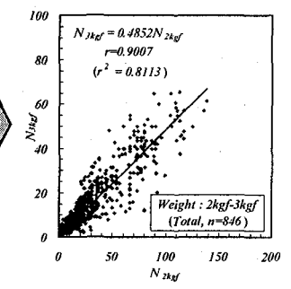
(c) N_{2kgf} と N_{3kgf} との関係
