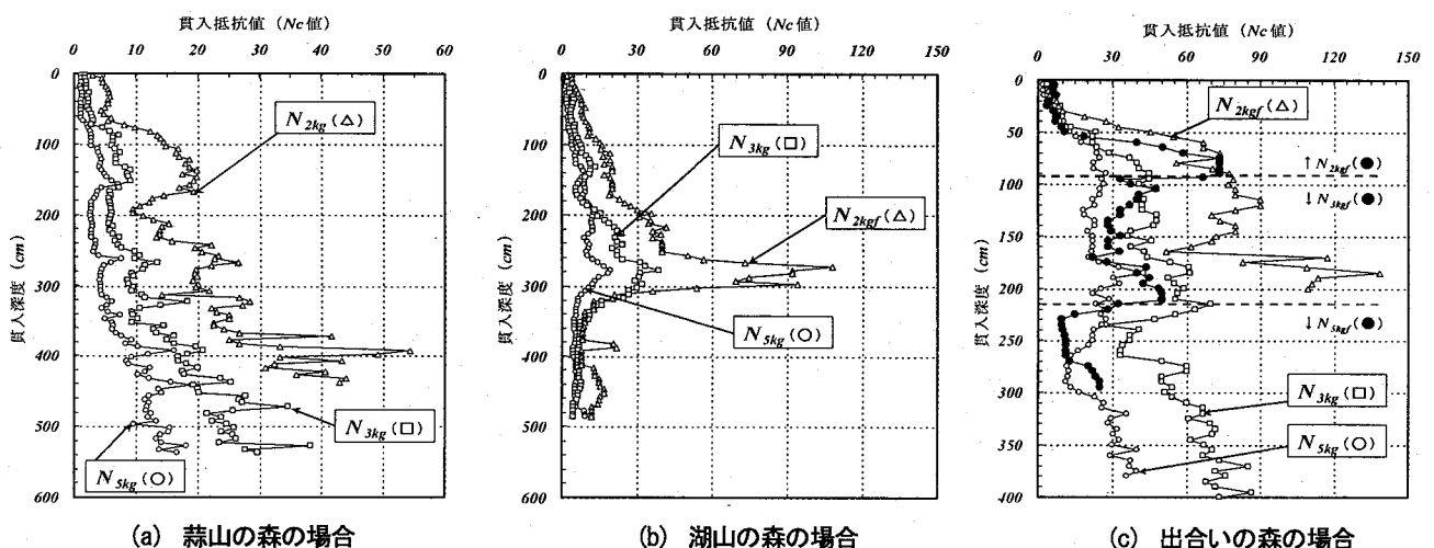
図-1 貫入抵抗値の深度分布の一例
