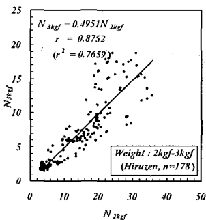
(c) N_{2kgf} と N_{3kgf} との関係
