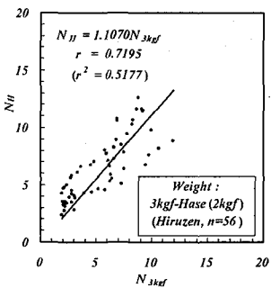
(d) N_{3kgf} と N_H との関係
