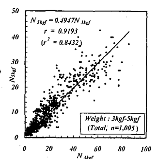
(a) N_{3kgf} と N_{5kgf} との関係
