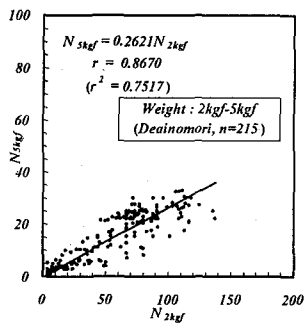
(b) N_{2kgf} と N_{5kgf} との関係
