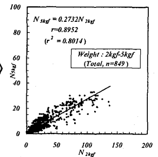
(b) N_{2kgf} と N_{5kgf} との関係
