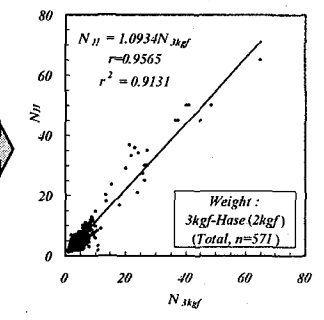
(d) N_{3kgf} と N_H との関係
