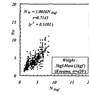
(d) N_{3kgf} と N_H との関係
