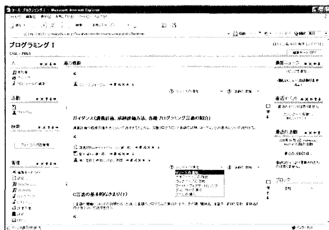
図-2 moodle「プログラミング」の Teacher 画面
