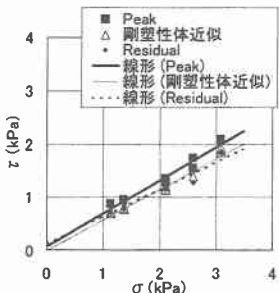
図 5 \tau - \sigma 線
