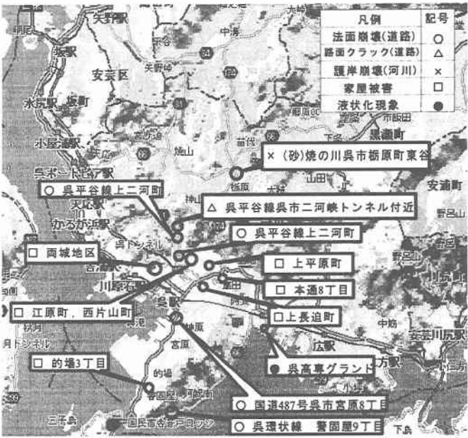
図 2 呉市の公共構造物と家屋被害
