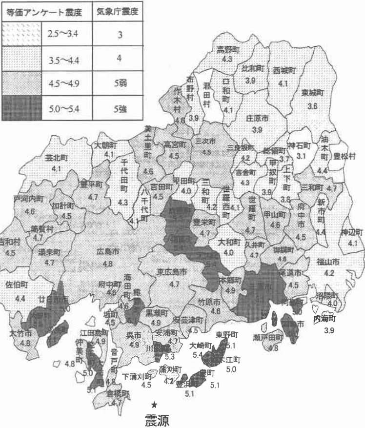
図 1 広島県の等価アンケート震度分布
